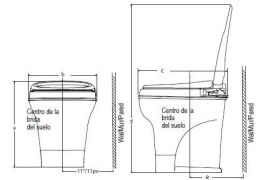
前视图
